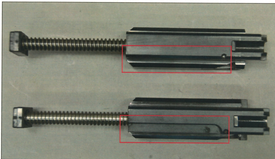
Abbildung 12: Ansicht Verschlussobenseite, oben der vollautomatische Verschluss „CZ Scorpion EVO 3 A1“, unten halbautomatische „CZ Scorpion EVO3 S1 Carbine C“ mit Ausnahme für quaderförmigen Einsatz
