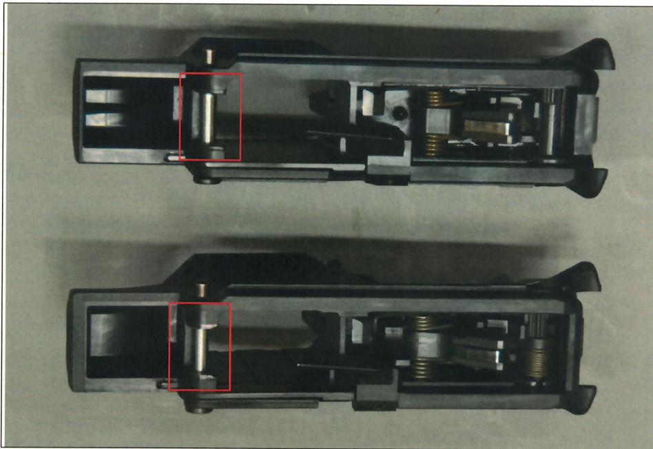
Abbildung 15: Ansicht Gehäuseunterteile mit unterschiedlich breiten Aufnahmen für das Abzugsmodul, oben „CZ Scorpion EVO 3 A1“, unten „CZ Scorpion EVO3 S1 Carbine C“ / „CZ Scorpion EVO3 S1 Carbine S“ / „CZ Scorpion EVO3 S1“
